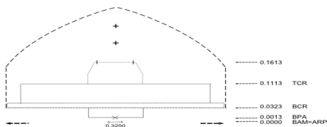
Esquema de antena
